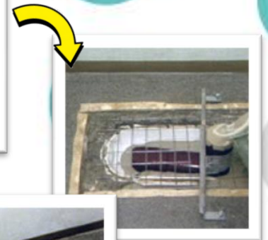
モルタルを打設 して埋め戻し
